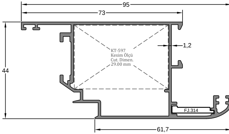
İçe Açılır Kanat Profili INWARD OPENING SASH PROFILE
