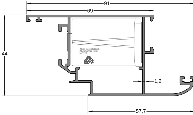
İçe Açılır Kanat Profili INWARD OPENING SASH PROFILE
